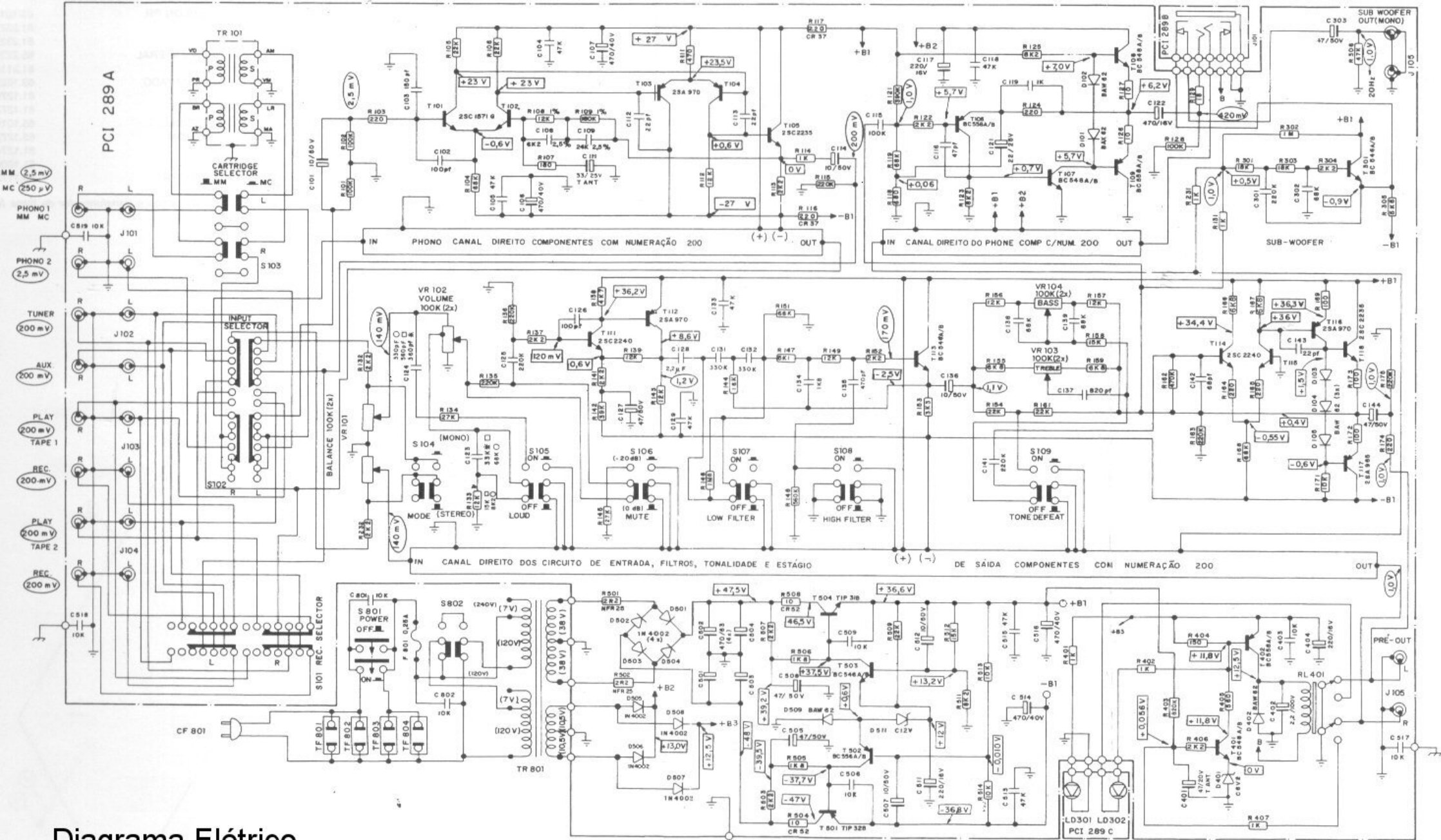
Diagrama Elétrico Stereo Control Pre-Amplifier P-II Gradiente
